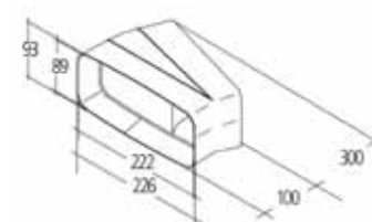
Bogen waagrecht 15°
