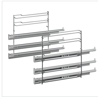
Teleskopvollauszug, 3-fach, Edelstahl HEZ638300
